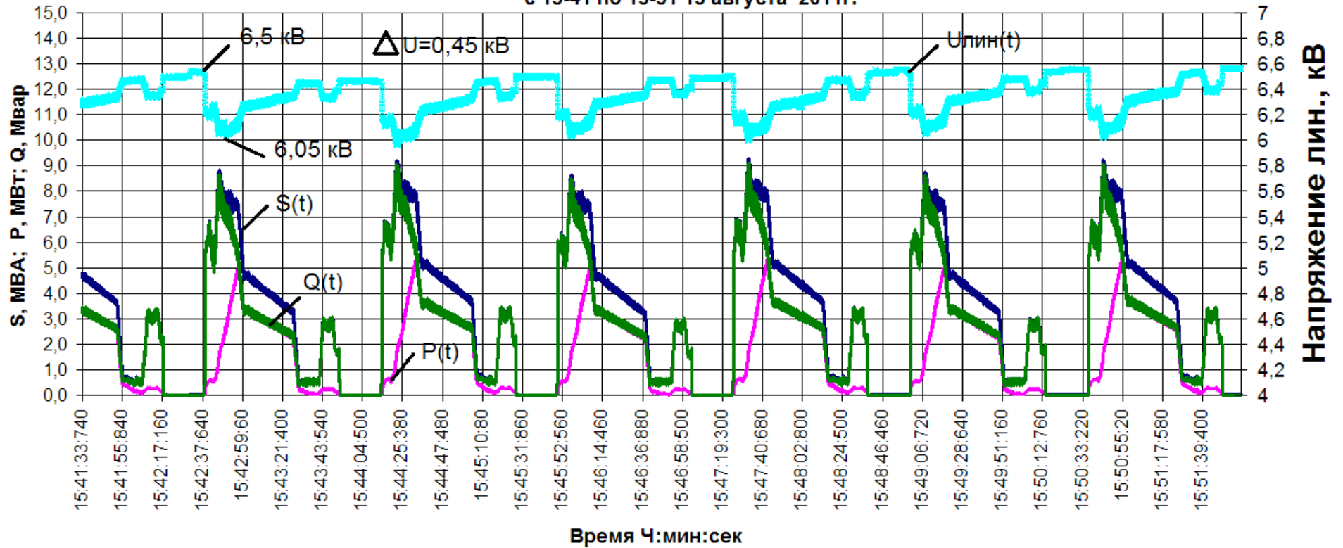
Графики полной, активной и реактивной мощностей потребления электроприводом шахтной подъемной машины и напряжения на шинах 6 кВ РП-2 БКПРУ-2.СТК (ФКУ) 12/6 отключен. с 15-41 по 15-51 15 августа 2011г.
