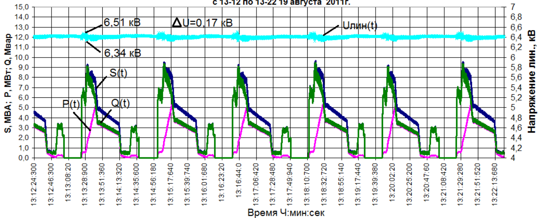
Графики полной, активной и реактивной мощностей потребления электроприводом шахтной подъемной машины и напряжения на шинах 6 кВ РП-2 БКПРУ-2. СТК (ФКУ) 12/6 включен. с 13-12 по 13-22 19 августа 2011г.
